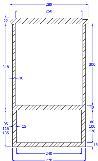
COUPE TRANSVERSALE
