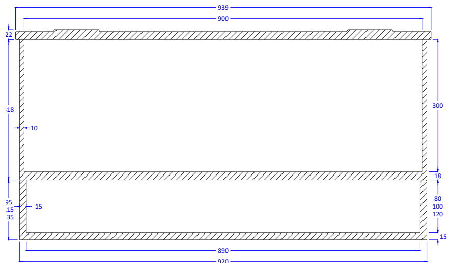
COUPE LONGITUDINALE
